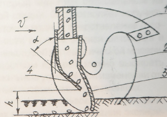
б) Рисунок 2 – Схема модернизированного узкорядного дискового сошника, а) вид спереди, б) вид сбоку: 1 – корпус; 2 – левый диск; 3 – профилеобразователь; 4 – рассеиватель
